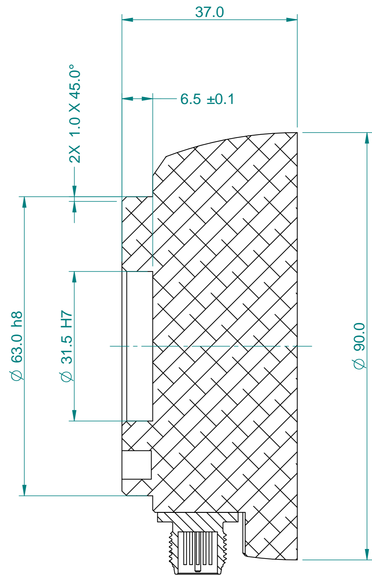
SECTION A-A
